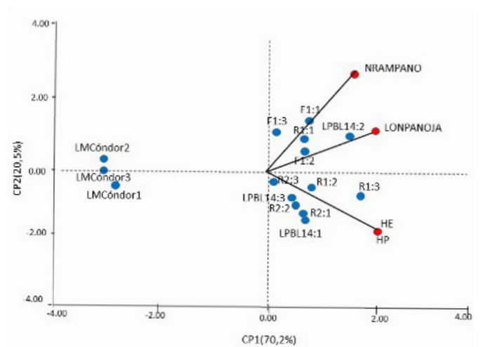
Figura 28. Biplot que resume la relación entre los genotipos y las variables altura de planta (HP), altura de inserción de espiga (HE), longitud de panoja (LONPANOJA), número de ramificaciones de la panoja (NRAMPANO) de la línea materna LM Cóndor y la línea paterna LP BLS14, la F 1 y las retrocruzadas (tres repeticiones de cada material)
