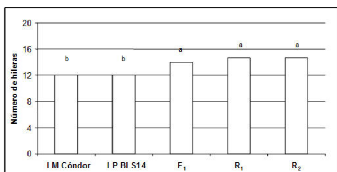
Figura 17. Número de hileras de granos de las líneas progenitoras LM Cónдор, LP BLS14, la F 1 y las retrocruzadas R 1 y R 2 . Letras distintas indican diferencias significativas al 5% con el test de Tukey.
