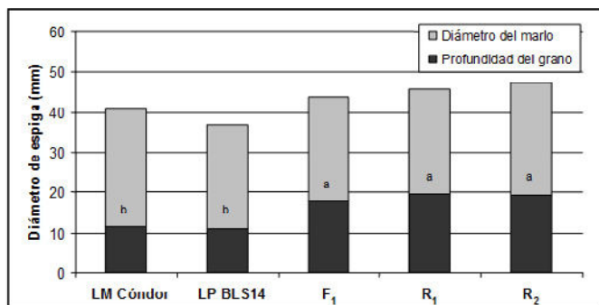
Figura 18. Profundidad del grano (mm) obtenida por diferencia entre el diámetro de espiga y diámetro del marlo de las líneas progenitoras LM Cónдор y LP BLS14, la F 1 y las retrocruzadas R 1 y R 2 . Letras distintas indican diferencias significativas al 5% con el test de Tukey.
