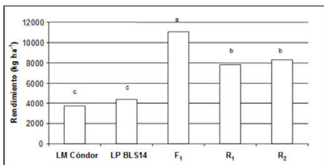
Figura 13. Rendimiento en grano (kg ha -1 ) de las líneas progenitoras LM Cónдор, LP BLS14, la F 1 y las retrocruzadas R 1 y R 2 (LM= Línea materna; LP= Línea paterna). Letras distintas indican diferencias significativas al 5% con el test de Tukey.
