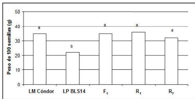
Figura 16. Peso de 100 semillas (g) de las líneas progenitoras LM Cónдор, LP BLS14, la F 1 y las retrocruzadas R 1 y R 2 . Letras distintas indican diferencias significativas al 5% con el test de Tukey.
